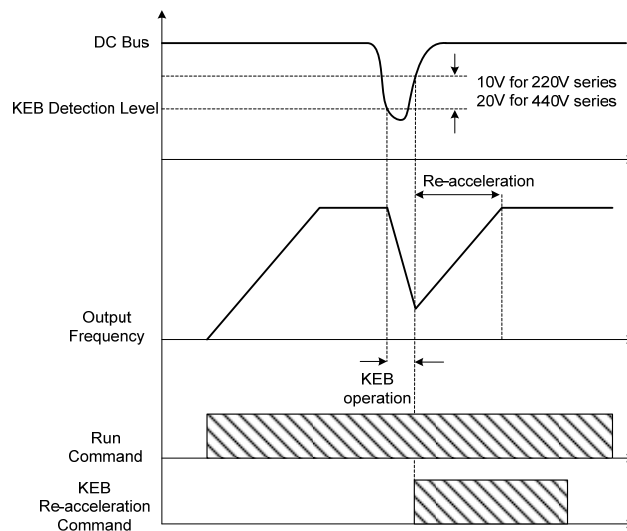
圖 4.3.82 KEB 操作
