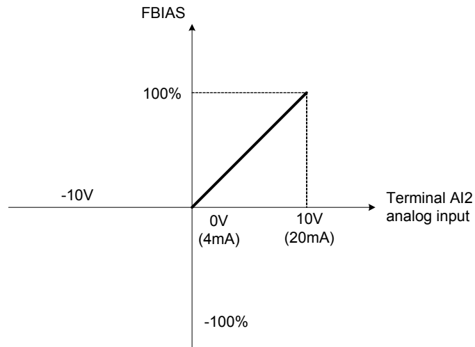
圖4.3.30 偏壓調整
