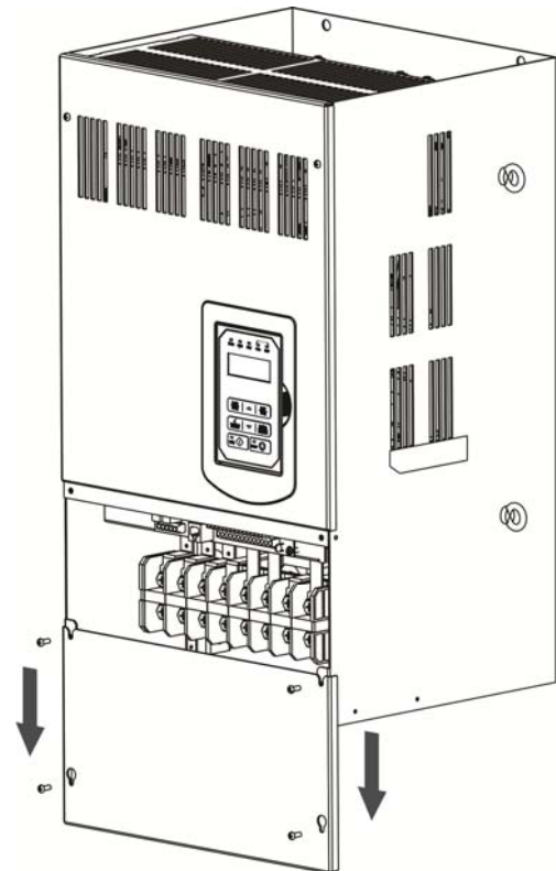
步驟二：拆卸端子外蓋
