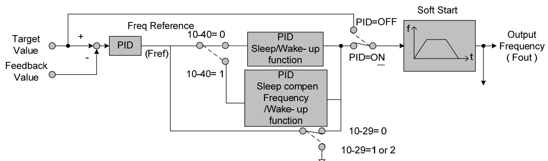
(a) PID 控制方塊圖
