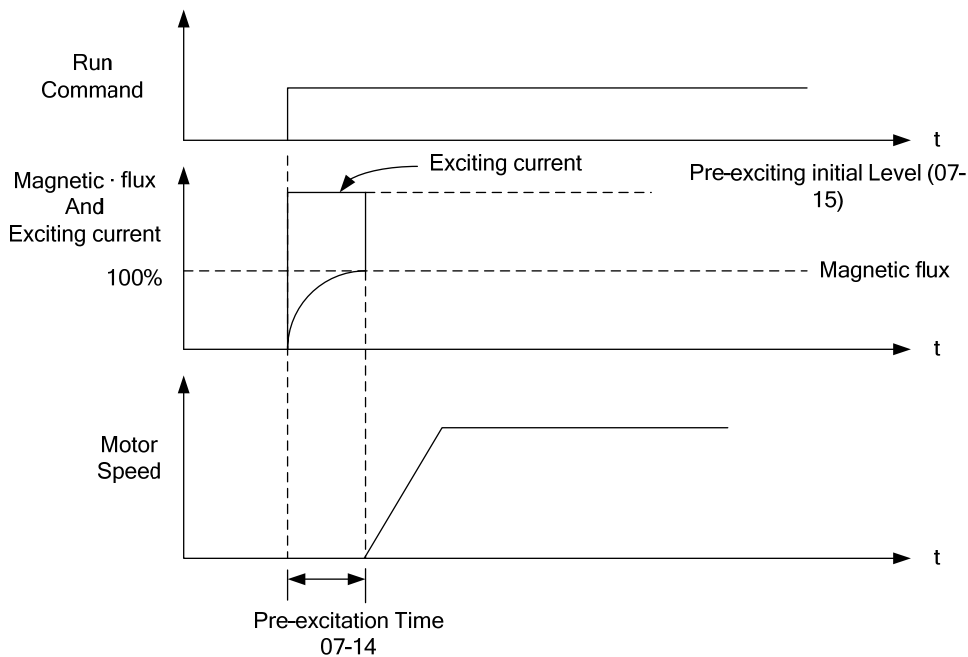
圖4.3.52 預激磁操作
