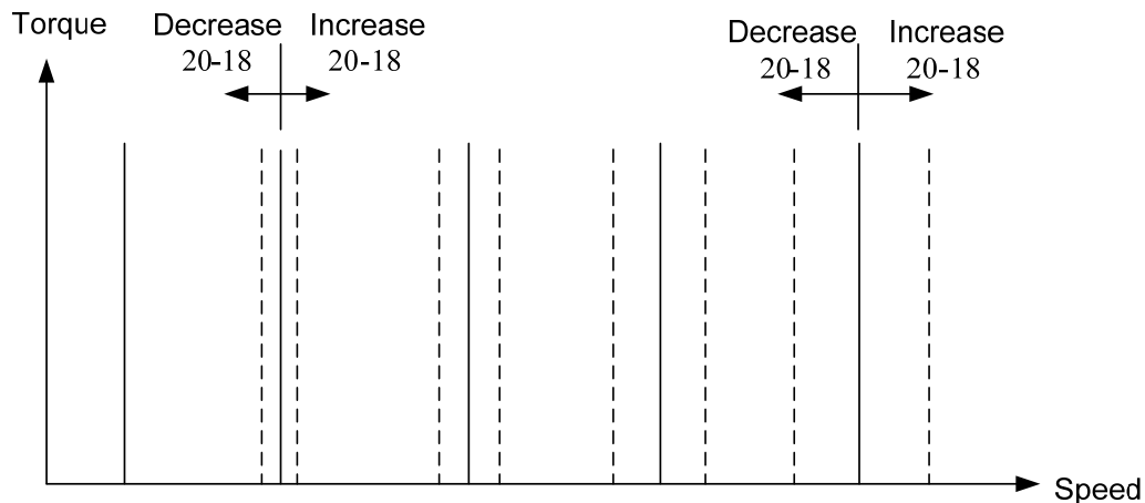
圖 4.3.99 20-18 對於轉矩-速度曲線的影響
