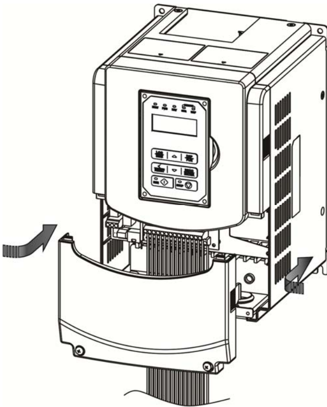
步驟三：裝配線路後，並裝回端子外蓋
