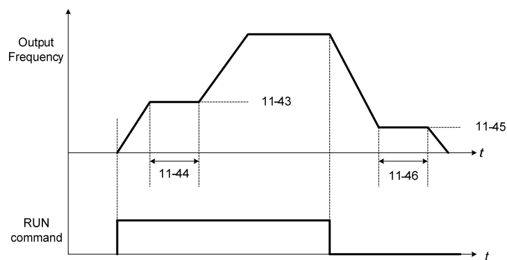
圖 4.3.81 保持功能
