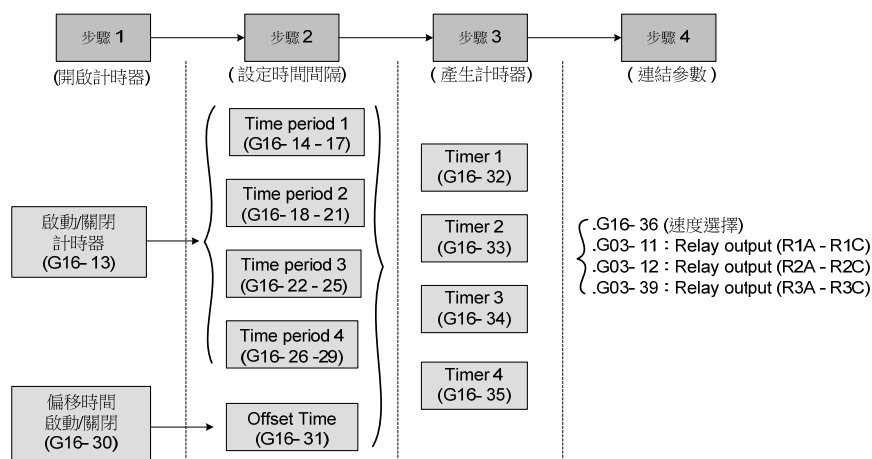
圖 4.3.85 RTC 架構
