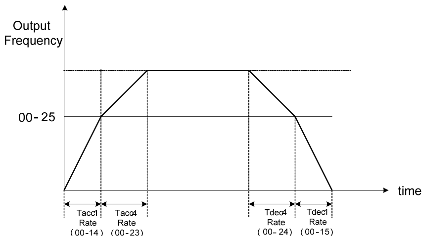
圖 4.3.8 自動加/減速交換
