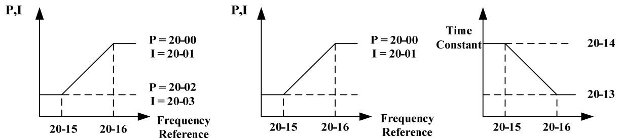
圖 4.3.116 SLV 模式之 ASR 增益設定
