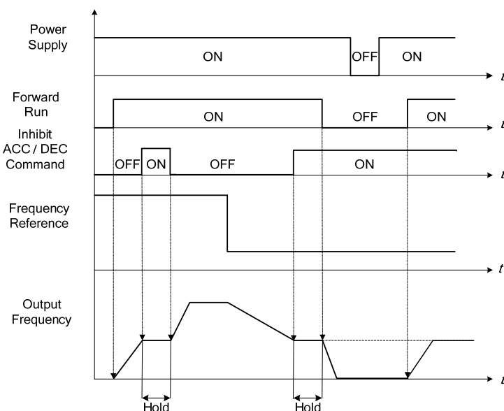
圖 4.3.21 加/減速禁止操作方式
