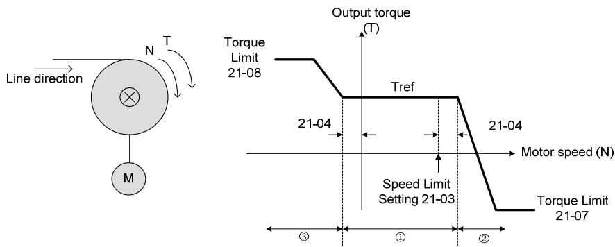
圖 4.3.128 捲繞操作
