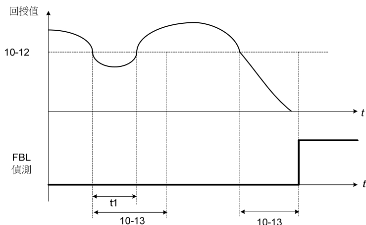
圖 4.3.83 PID 回授斷線偵測
