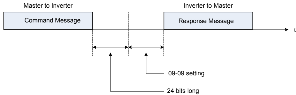
圖 4.3.77 訊息空間
