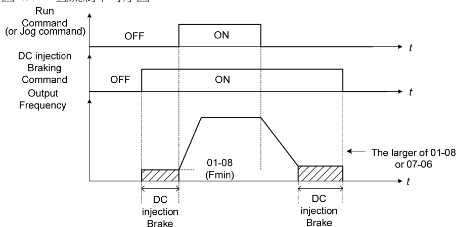
圖 4.3.24 直流剎車時序圖
