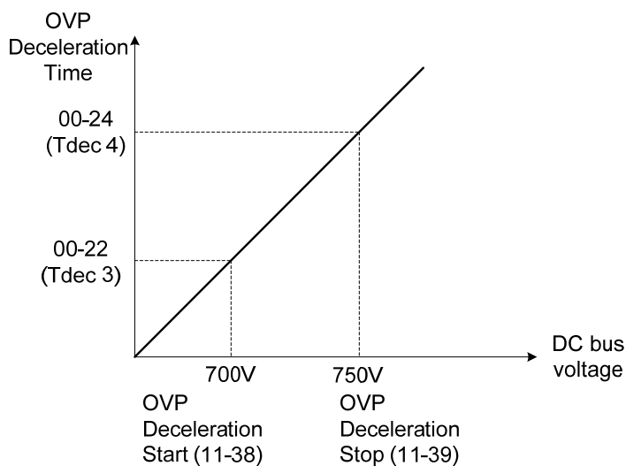
圖 4.3.93 OVP減速時間
