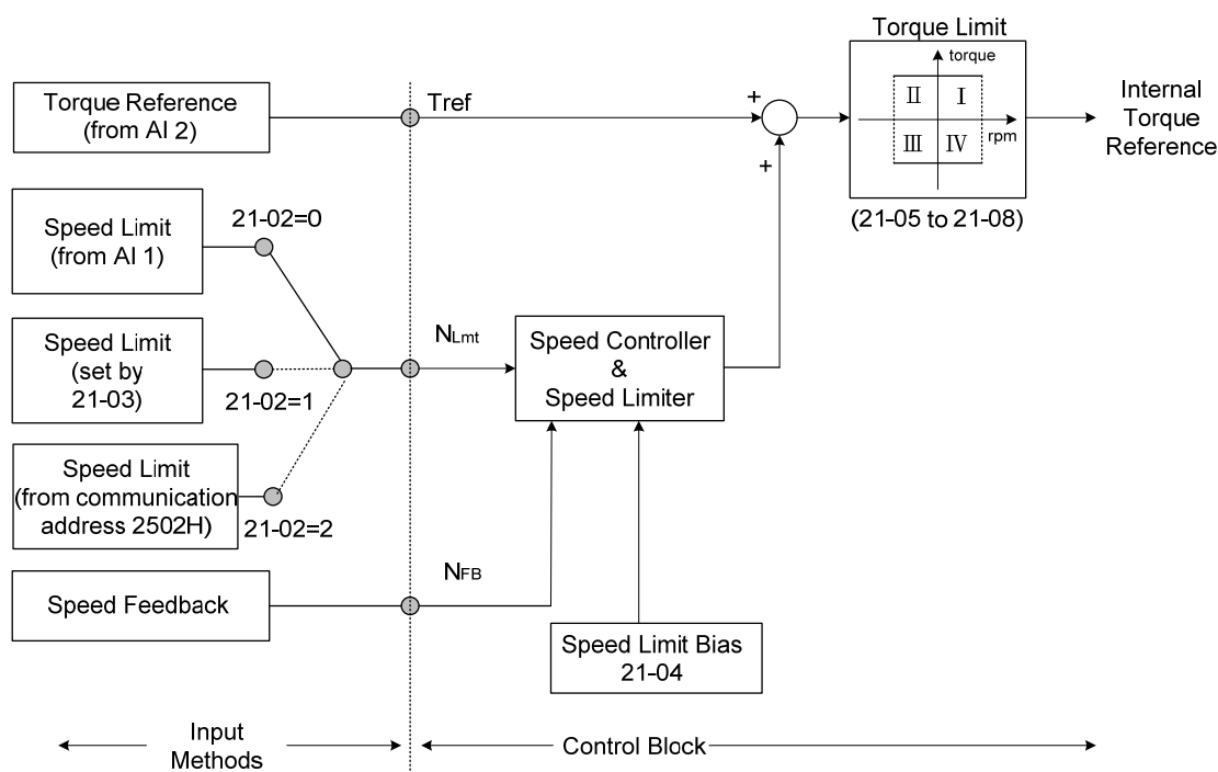
圖 4.3.125 轉矩控制方塊圖
