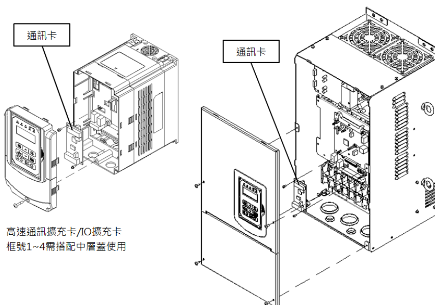
通訊卡安裝示意圖
