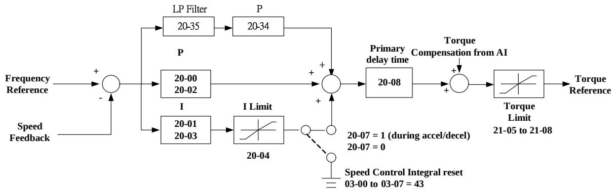
4.3.113 速度控制架構(SV 模式及 PMSV 模式)
