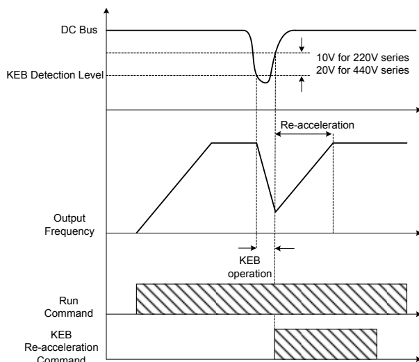
圖 4.3.96 KEB 操作
