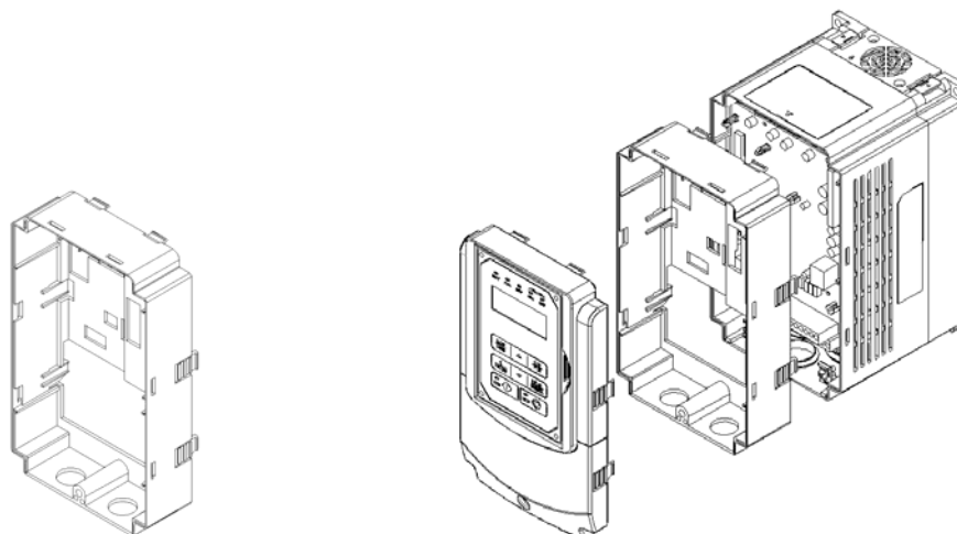
中層蓋外觀圖
