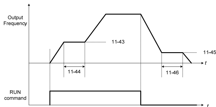
圖 4.3.95 保持功能
