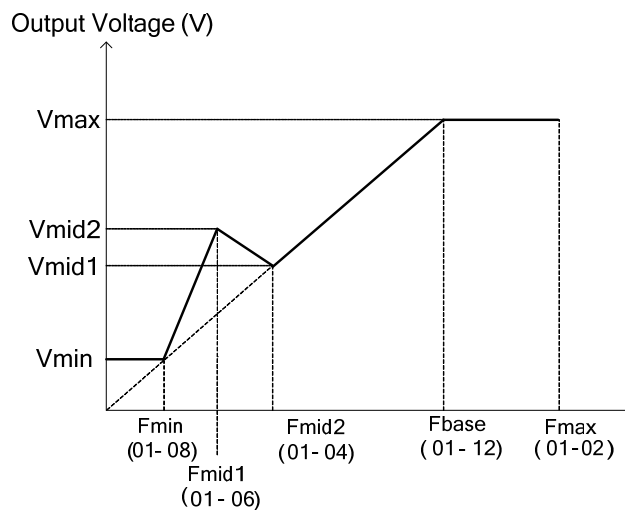
圖 4.3.13 轉矩提升
