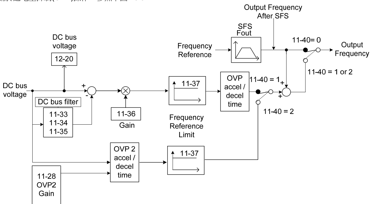
圖 4.3.92 OVP操作
