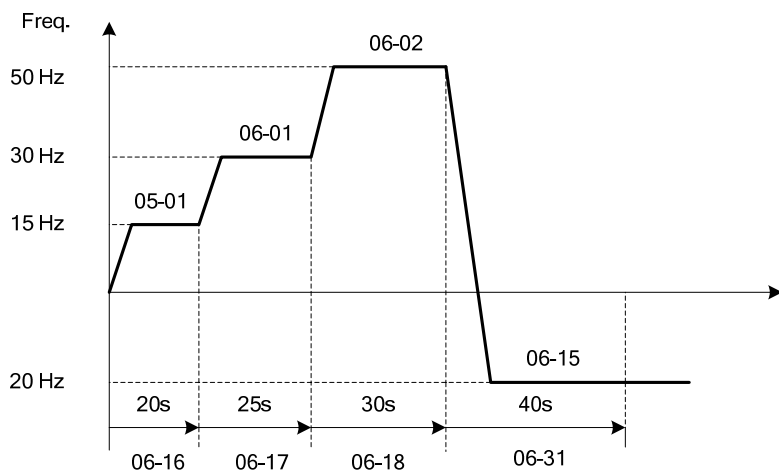
圖 4.3.54 單循環的自動運轉(持續)
