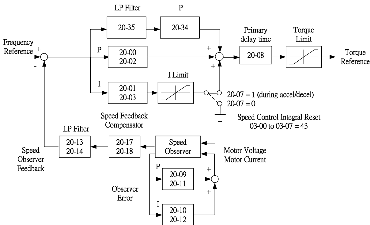
圖 4.3.112 速度控制架構(SLV 模式)
