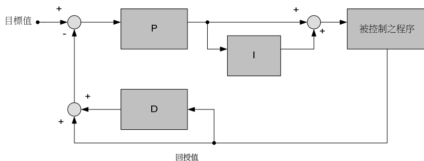
圖 4.3.79 回授微分值 PID 控制
