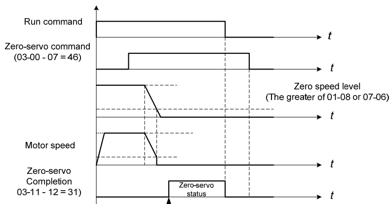
圖 4.3.97 零伺服操作
