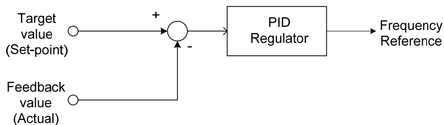
圖 4.3.28 PID控制
