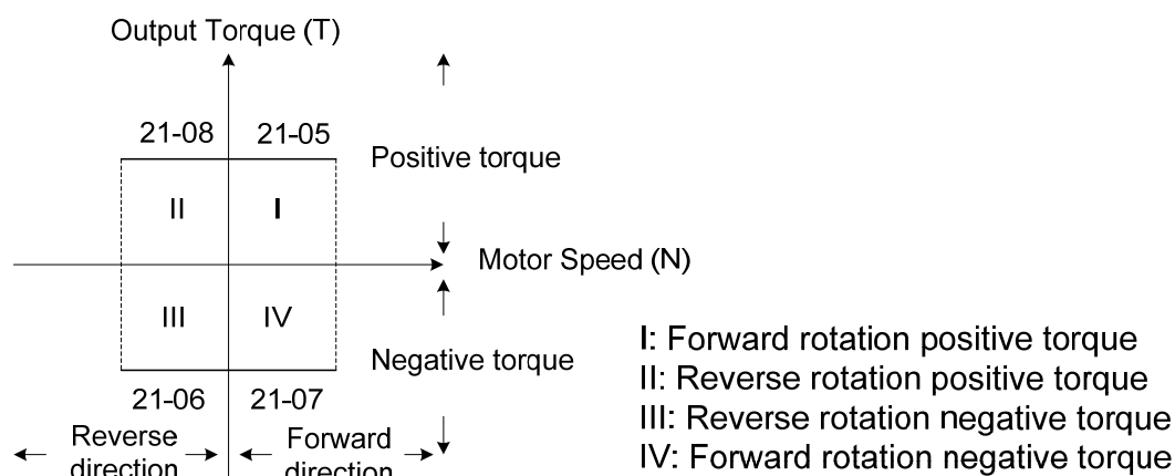
圖 4.3.131 四象限之轉矩限制設定
