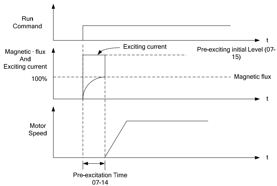
圖4.3.62 預激磁操作
