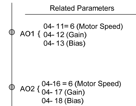
圖 4.3.115 類比輸出設定
