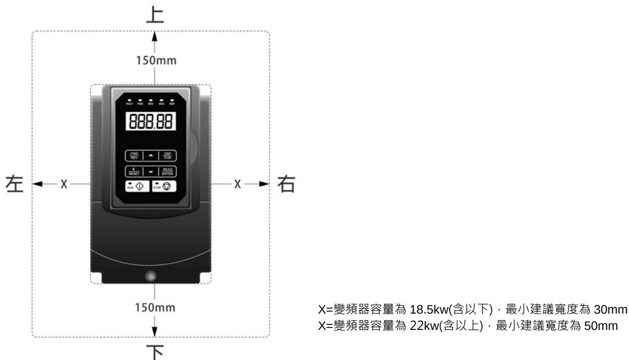
圖 3.1 A510s 的安裝空間
