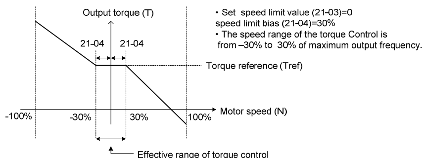
圖 4.3.126 速度限制設定
