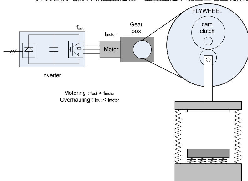
圖 4.3.91 沖壓操作
