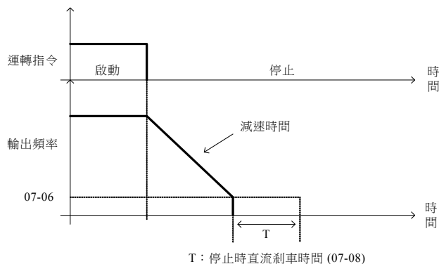
圖 4.3.58 減速停止
