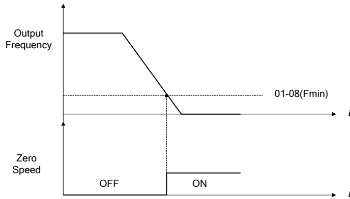
圖4.3.26 零速度操作
