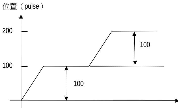
圖 4.3.135 絕對型示意圖
