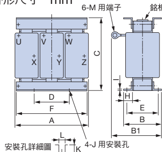
外觀圖1
