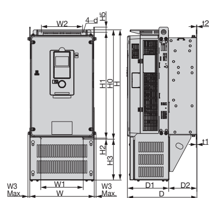
外觀圖 3
