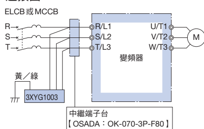
連接圖
