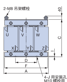
外觀圖3
