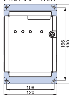
外形尺寸 mm
