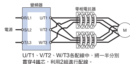
連接圖c
