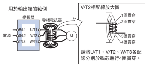
連接圖a
