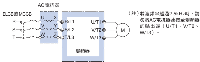
連接圖
