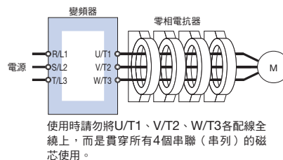
連接圖b
