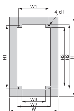
面板加工圖1
