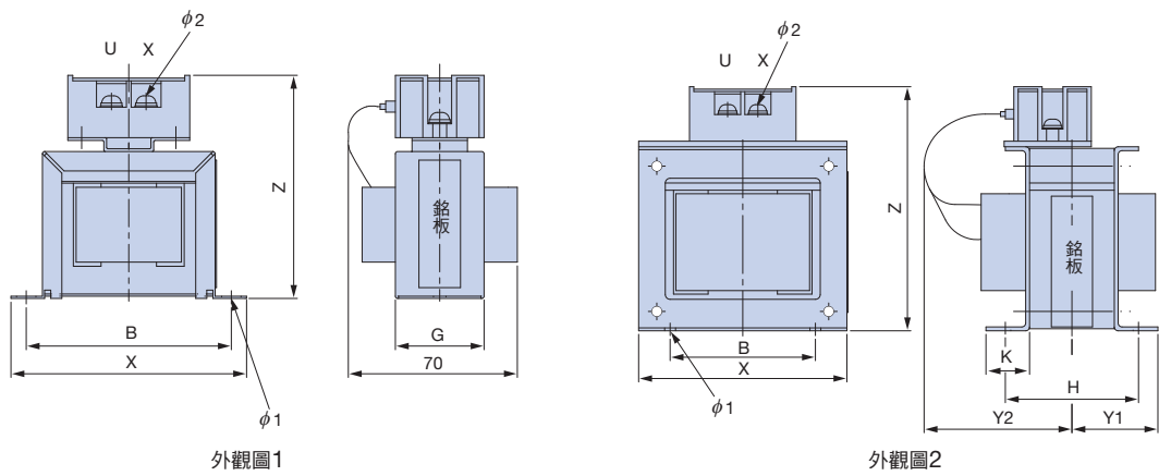
外形尺寸 mm
