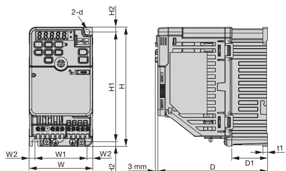
外觀圖 1
