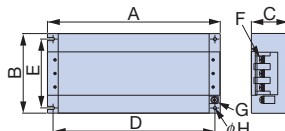
外觀圖3
