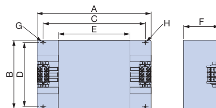
外觀圖2
