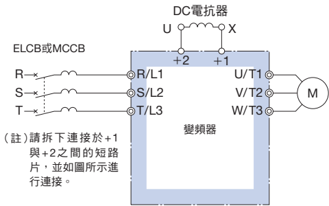
連接圖
