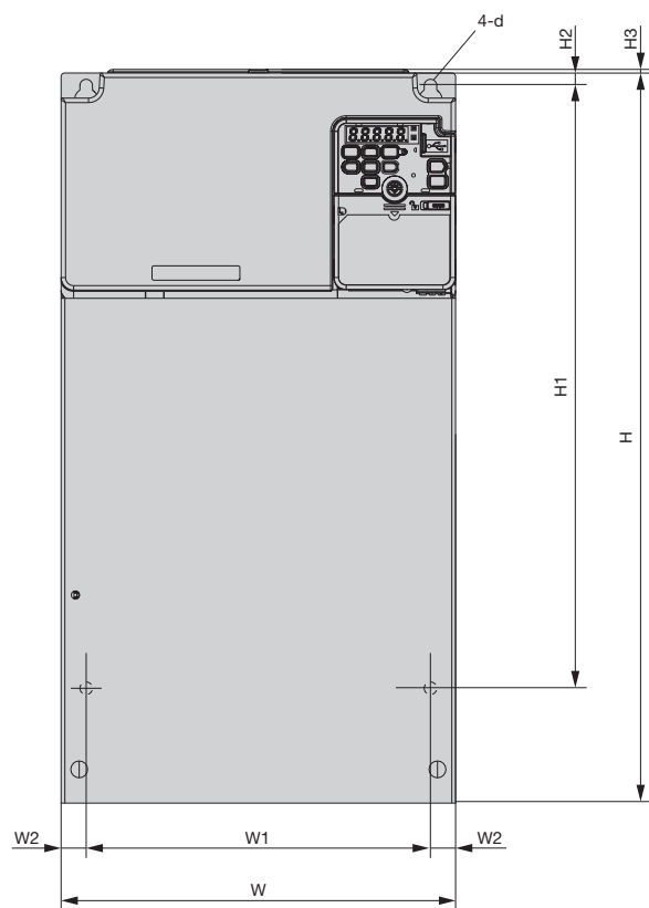
外觀圖 3
