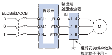
連接圖
