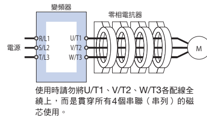
連接圖b
