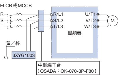
連接圖
