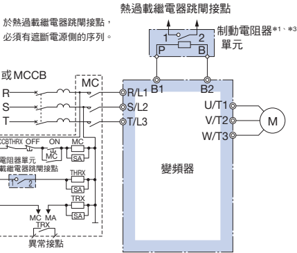
連接圖B
