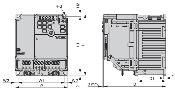
外觀圖 2
