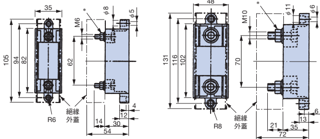
外觀圖1
