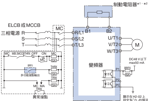
連接圖A
