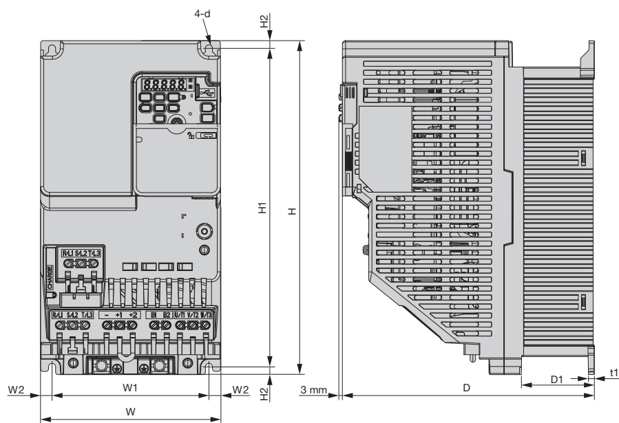
外觀圖 3
