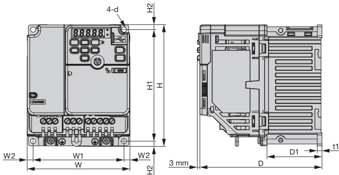
外觀圖 2
