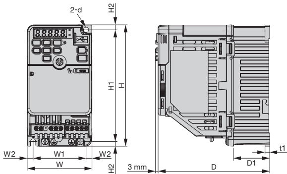
外觀圖 1
