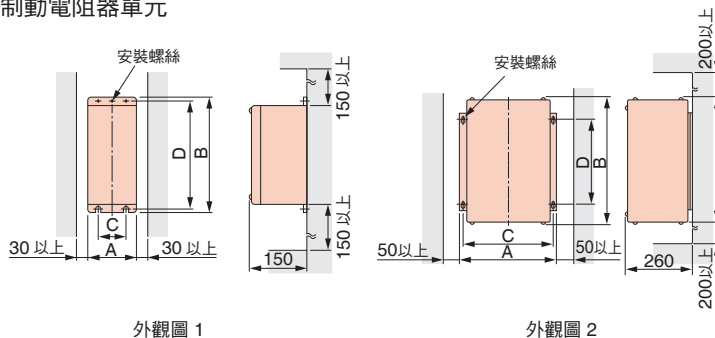
外觀圖 1
