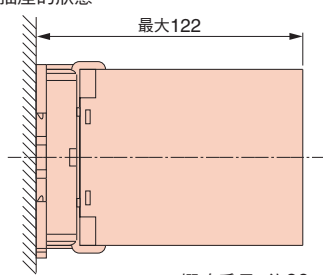
已安裝插座的狀態
