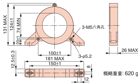
型號 F11080GB
