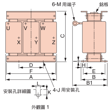
外觀尺寸 mm
