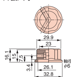
外觀尺寸 mm
