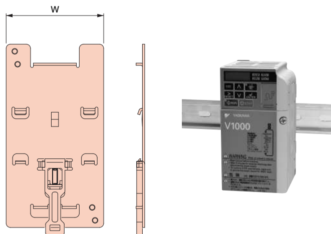
外觀尺寸（200 V、0.4 kW 範例）
