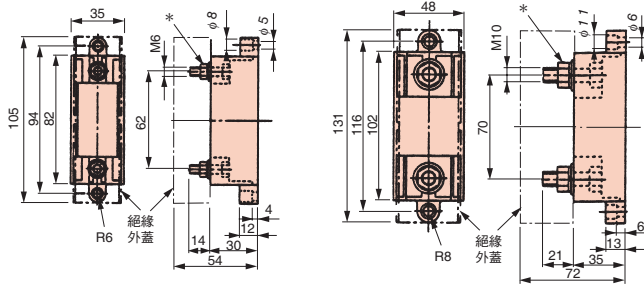
外觀圖 1
