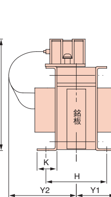
外觀圖 2
