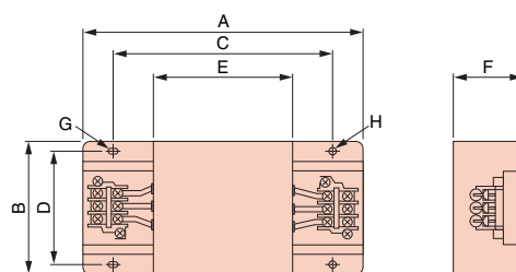
外觀尺寸 mm
