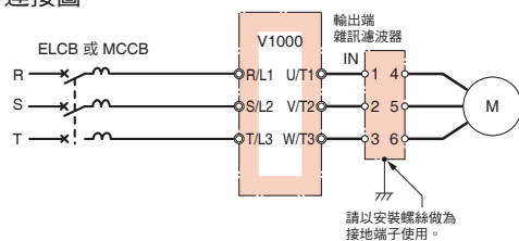
連接圖
