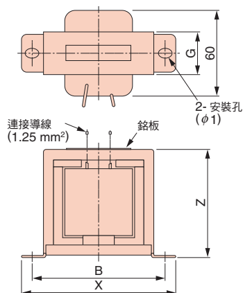
外觀尺寸 mm
