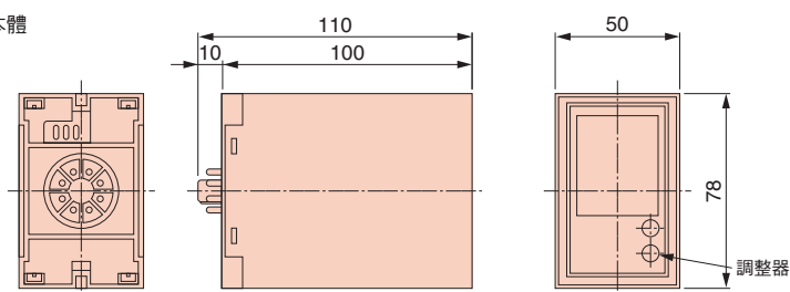
外觀尺寸 mm
