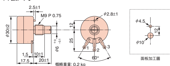
外觀尺寸 mm
