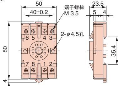
插座
