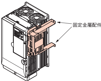
單元（PS-V10M）與固定金屬配件安裝完成時
