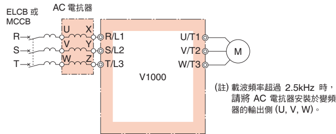
連接圖
