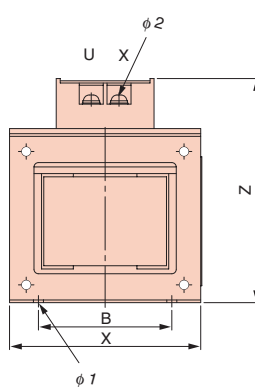
外觀圖 2
