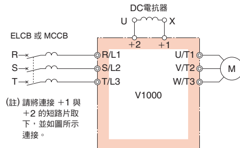
連接圖
