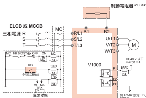
連接圖 A
