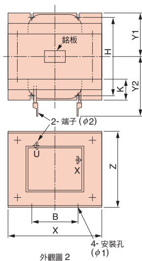
外觀圖 2
