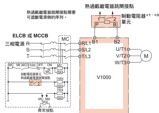
連接圖 B
