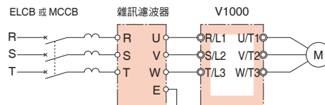
三相輸入時 (LNFD 型、FN 型)
