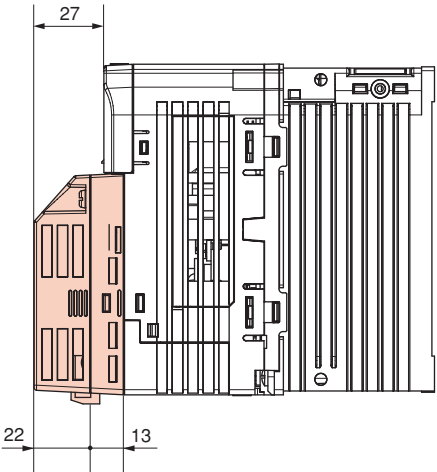
CIMR-VA2A0004 範例
