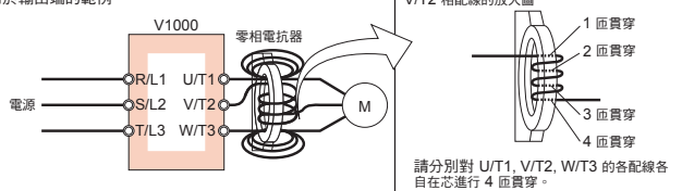
連接圖 a
