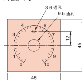
外觀尺寸 mm
