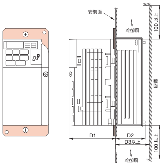
安裝尺寸圖（200 V、0.4 kW 範例）
