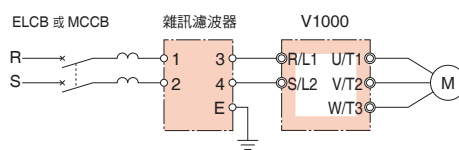
單相輸入時 (LNFB 型)
