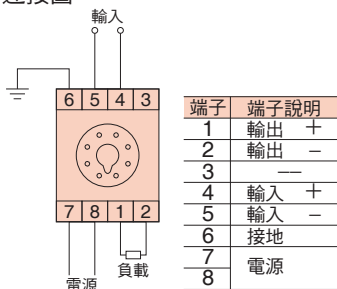
連接圖
