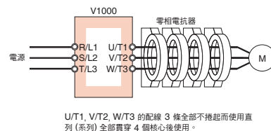
連接圖 b
