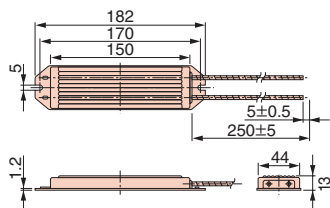
ERF-150WJ 系列
