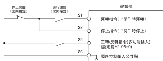
圖 3.2 3 線式控制
