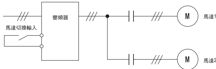
圖5.45 馬達的切換
