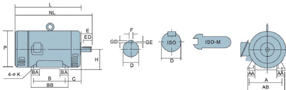
直流馬達外型圖(橫臥式)型 1HP-5HP尺寸圖
