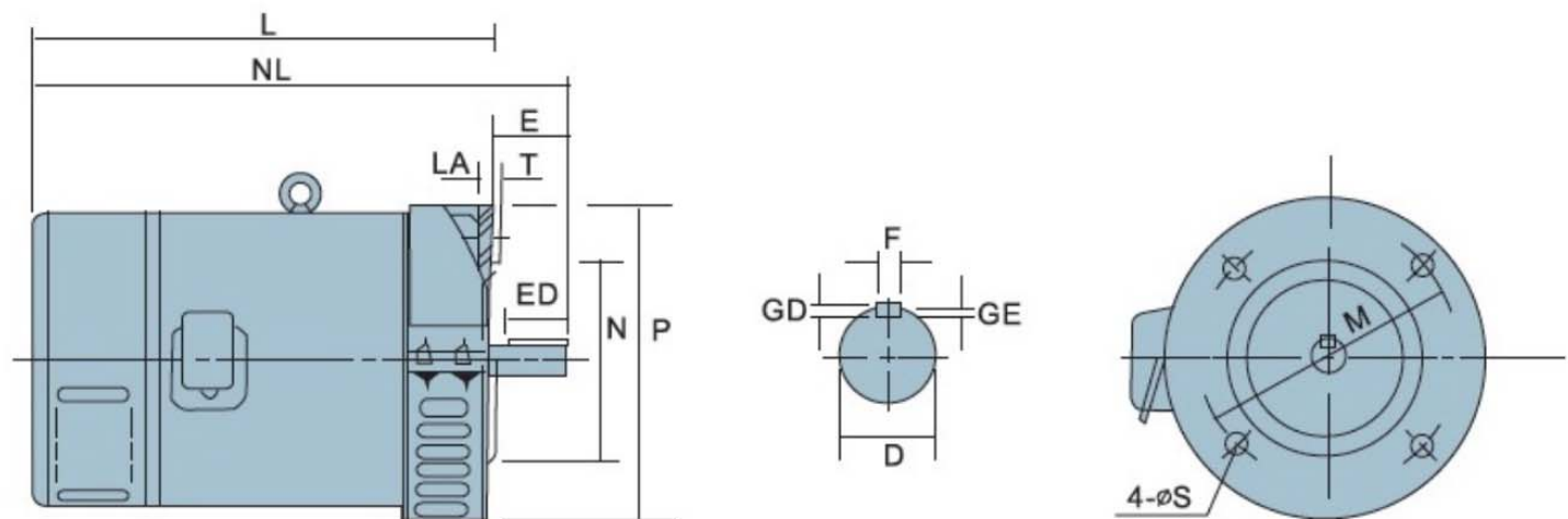
直流馬達外型圖(凸緣型/立式)TD型 1HP-3HP尺寸圖
