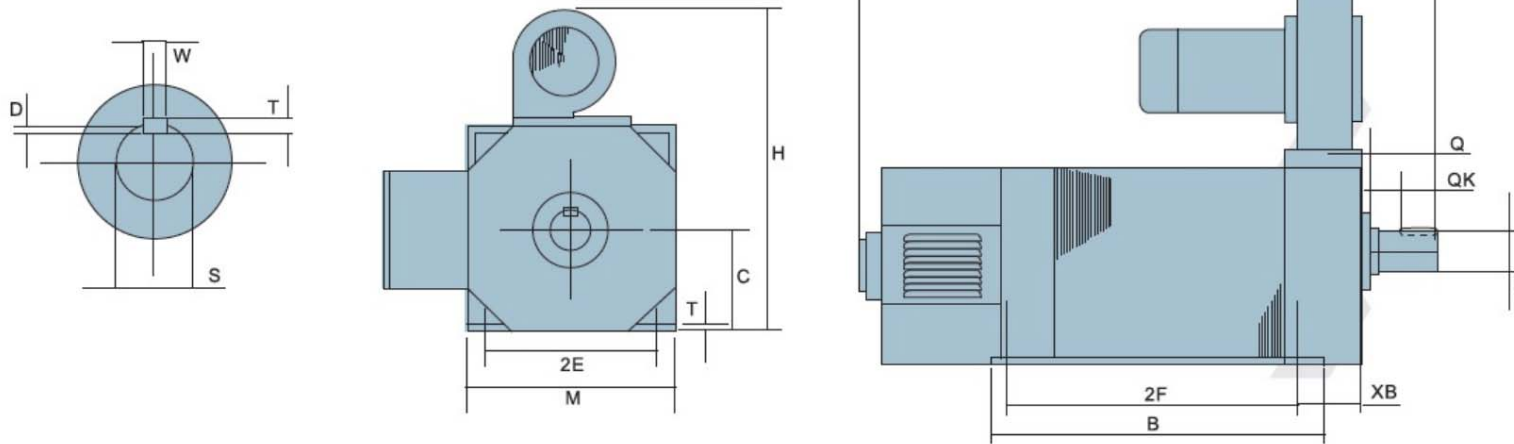
四方型歐規式馬達尺寸(積架式) 10HP-175HP尺寸圖
