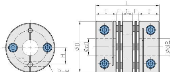
外徑 \phi 40 \sim \phi 65
