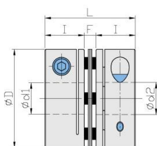
外徑 \phi 27 \sim \phi 34
