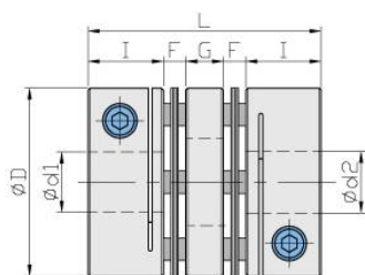
外徑 \phi 27 \sim \phi 34
