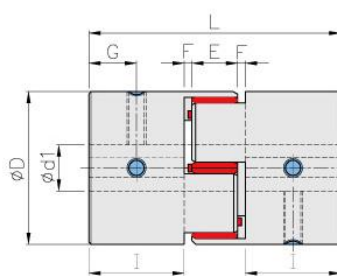
外徑 \phi 40 \sim \phi 65
